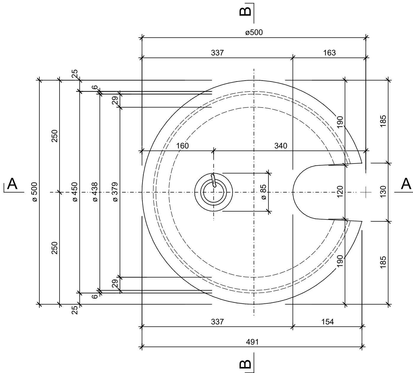
Grundriss, 1:5
