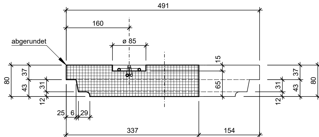
Schnitt A - A, 1:5
