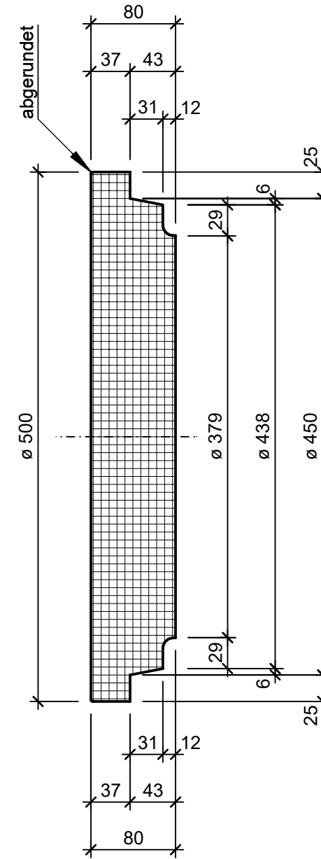
Schnitt B-B, 1:5
