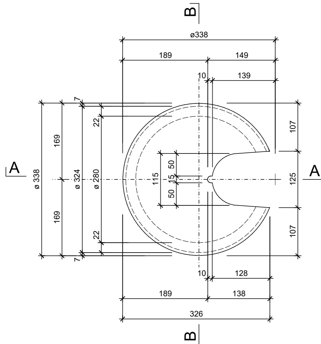
Grundriss, 1:5
