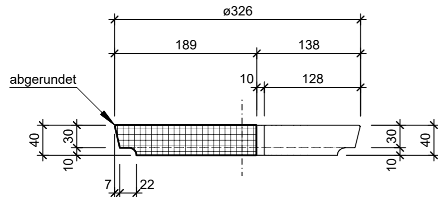
Schnitt A - A, 1:5
