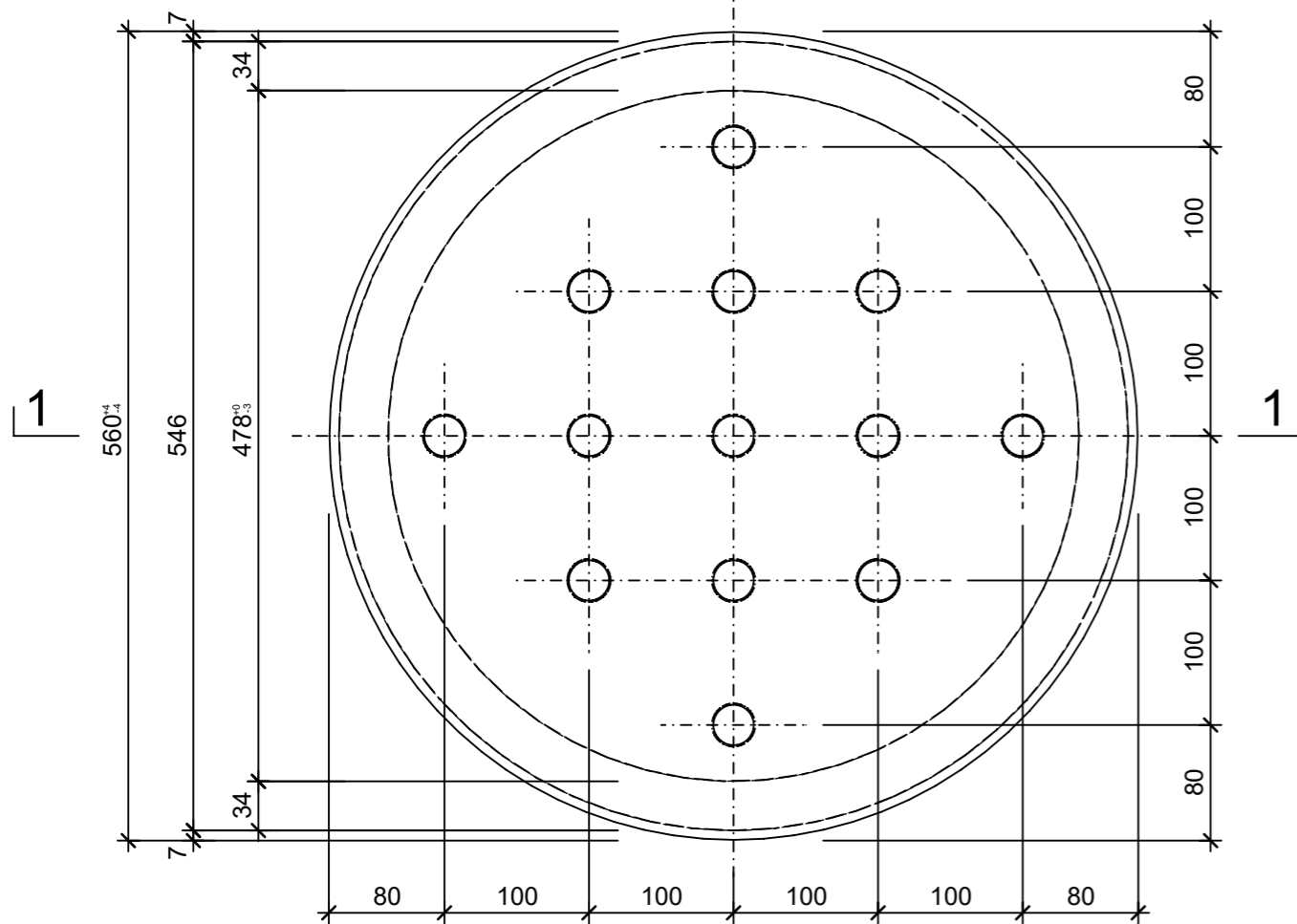
Grundriss, 1:5
