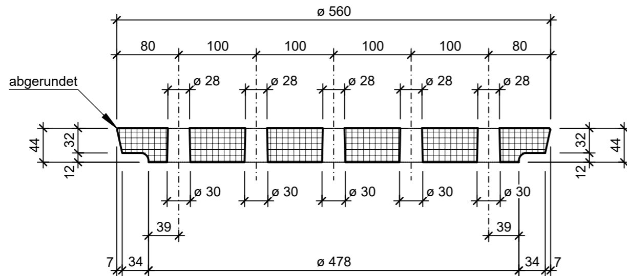
Schnitt A - A, 1:5
