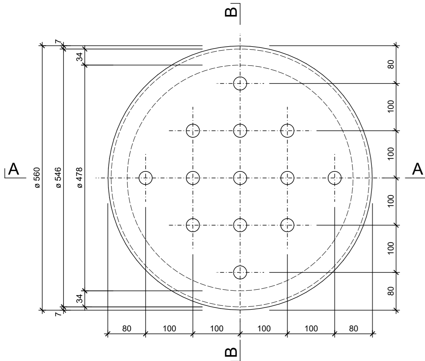
Grundriss, 1:5
