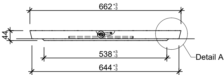
Schnitt 1-1, 1:10
