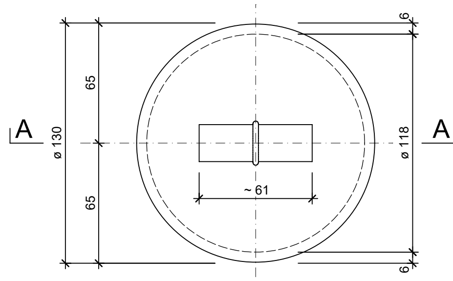
Grundriss, 1:2
