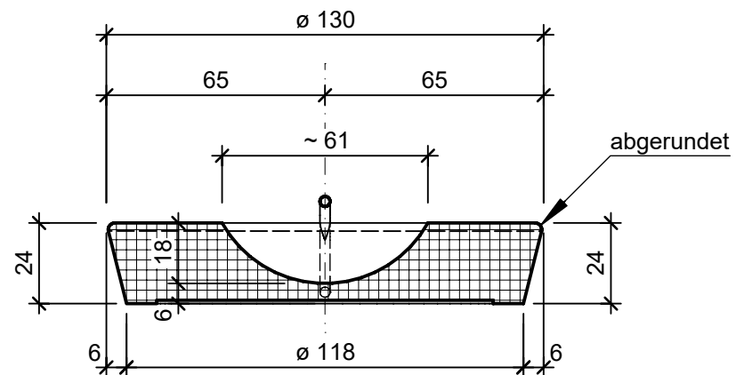
Schnitt A - A, 1:2
