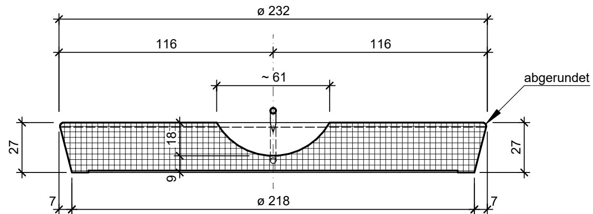
Schnitt A - A, 1:2
