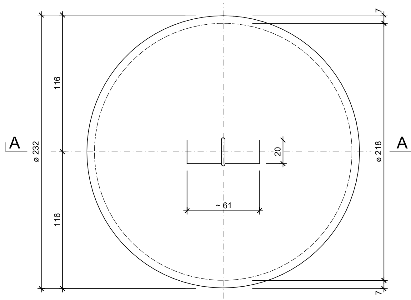
Grundriss, 1:2
