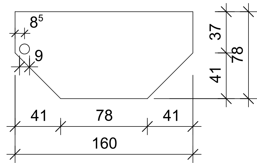
Grundriss, 1:2
