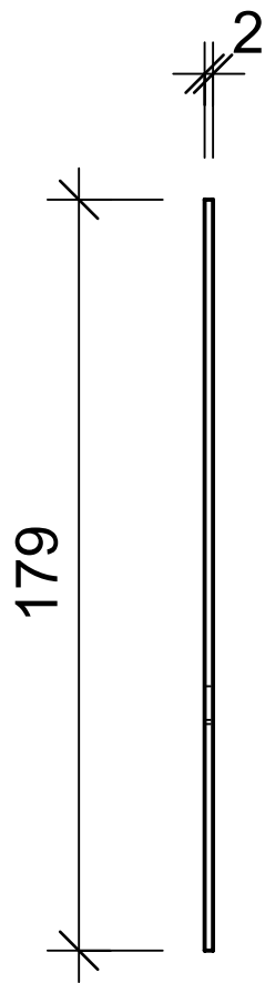
Schnitt 2-2, 1:2
