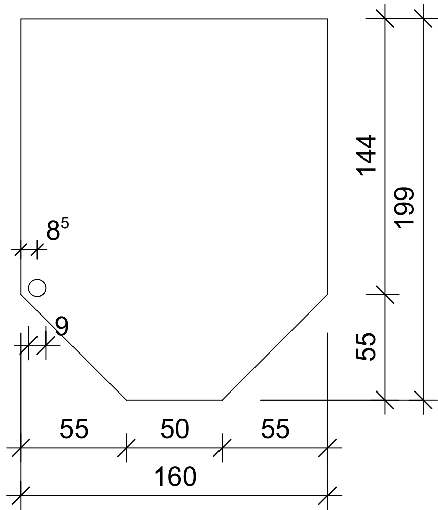
Ansicht 1-1, 1:2
