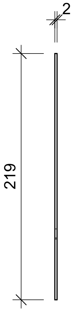
Schnitt 2-2, 1:2
