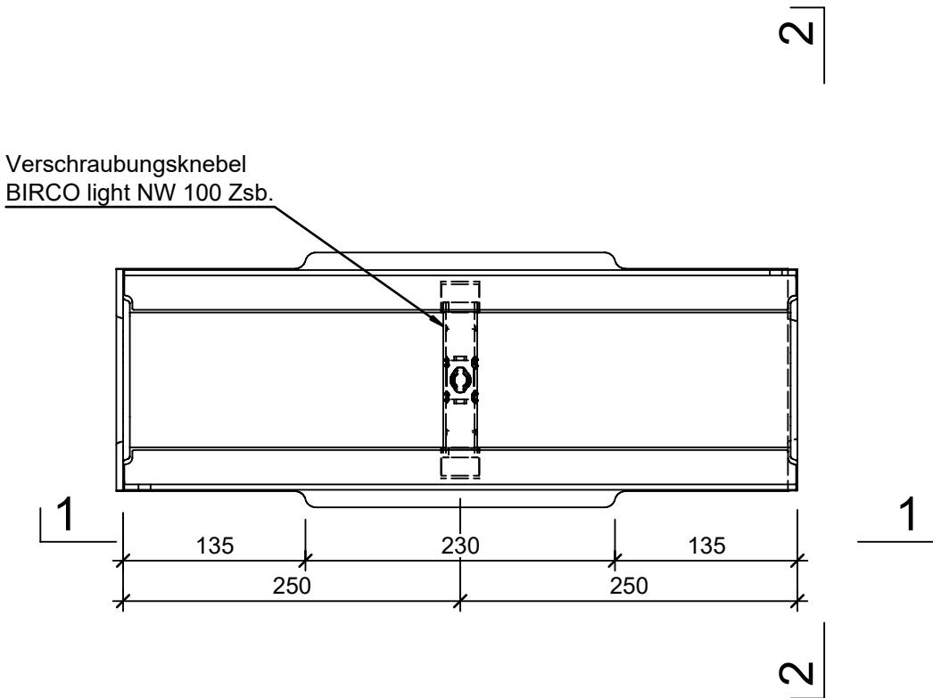
Grundriss, 1:5
