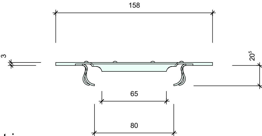
Isometrie
