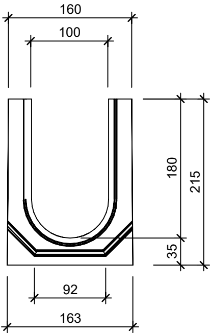
Schnitt 2-2, 1:5 Feder
