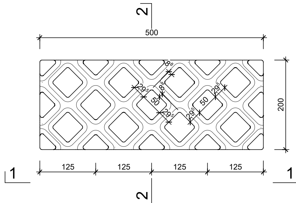
Grundriss 1:5
