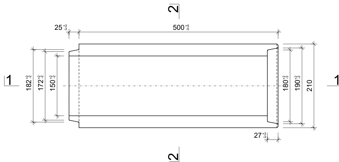
Grundriss, 1:5
