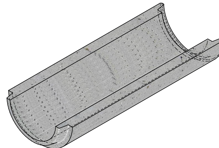
Isometrie, 1:5
