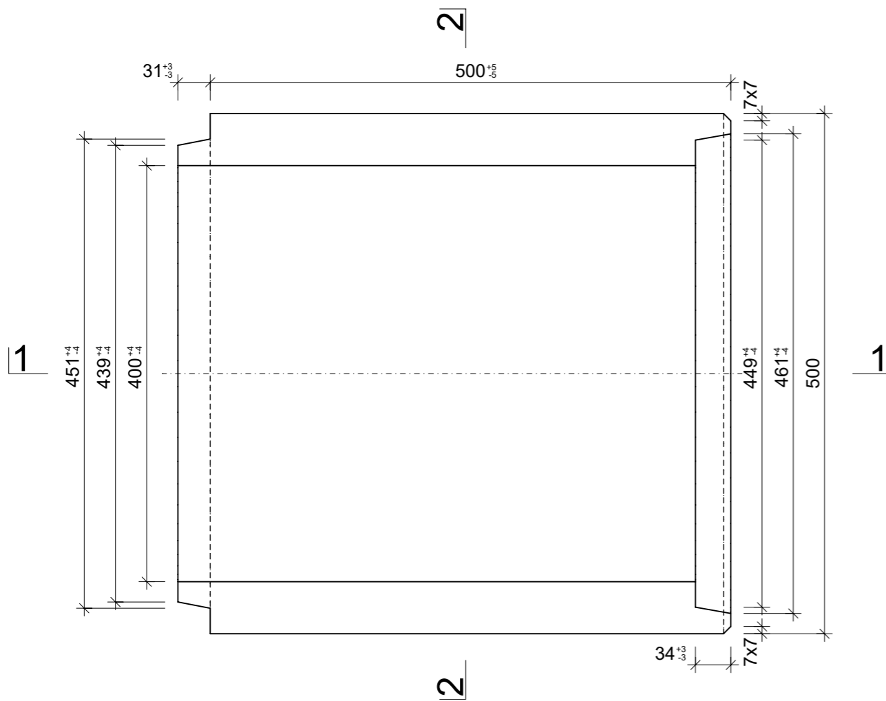
Grundriss, 1:5
