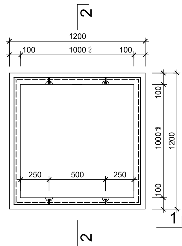
Grundriss, 1:20
