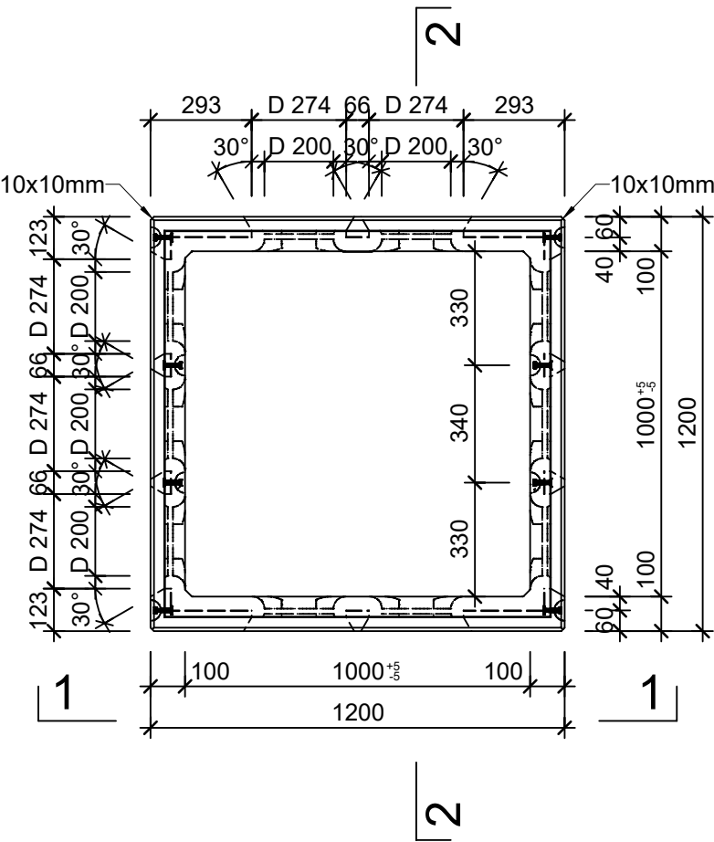
Grundriss, 1:20
