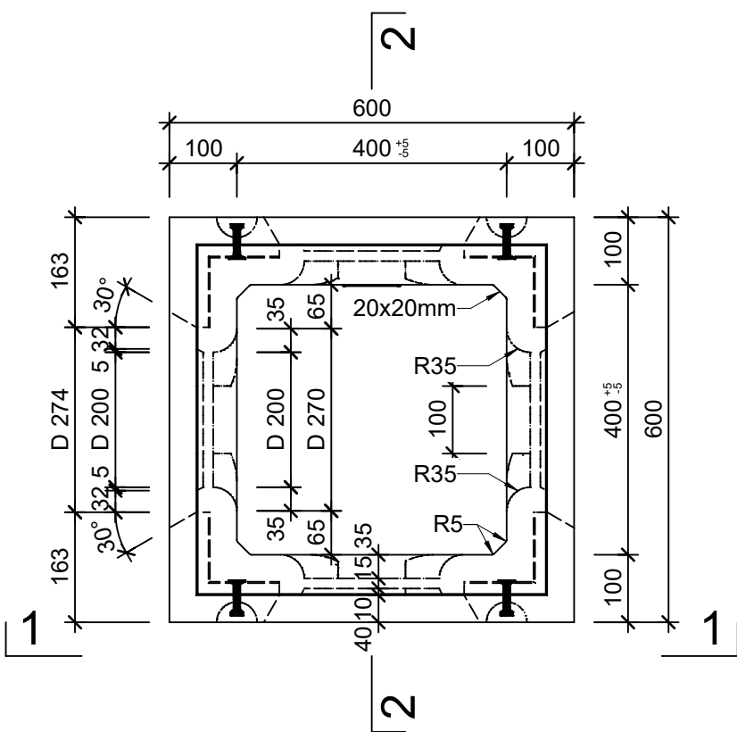
Grundriss, 1:10
