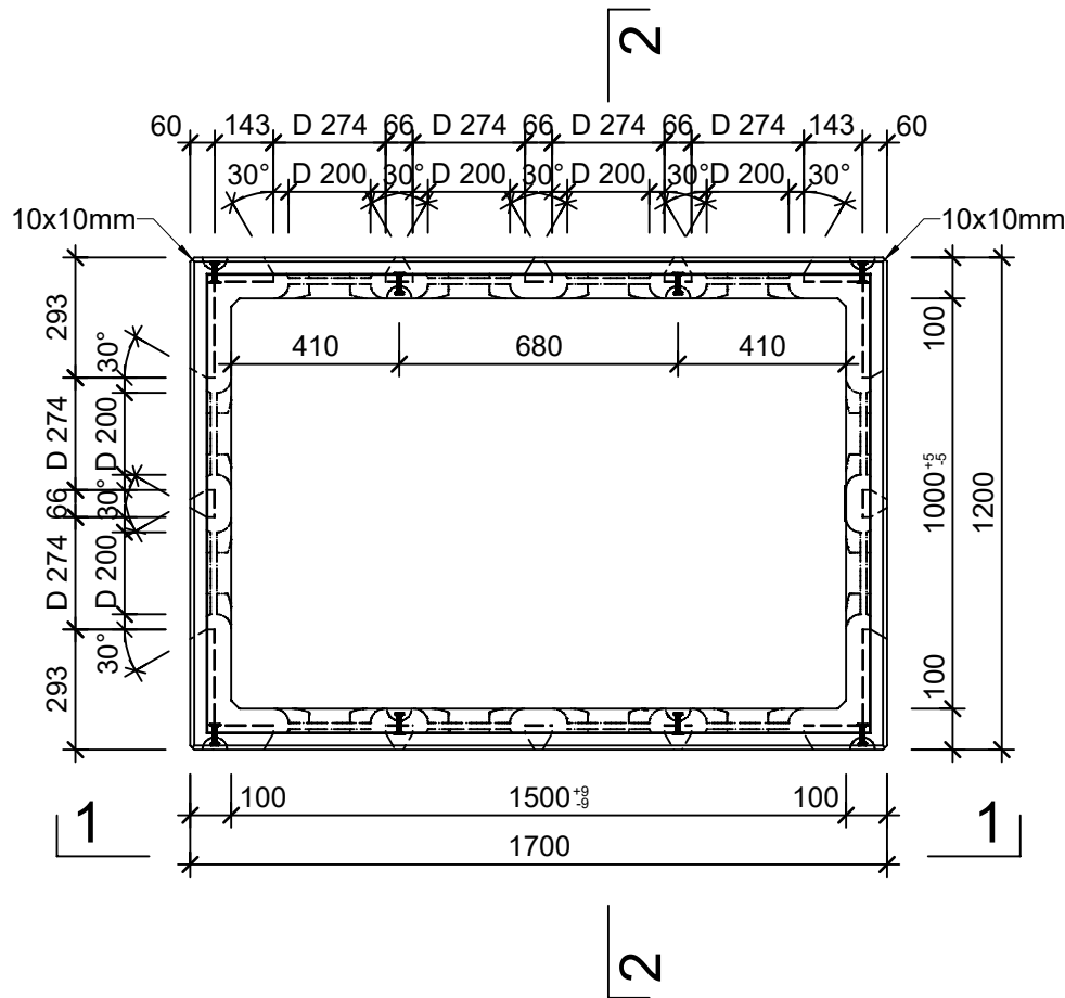
Grundriss, 1:20
