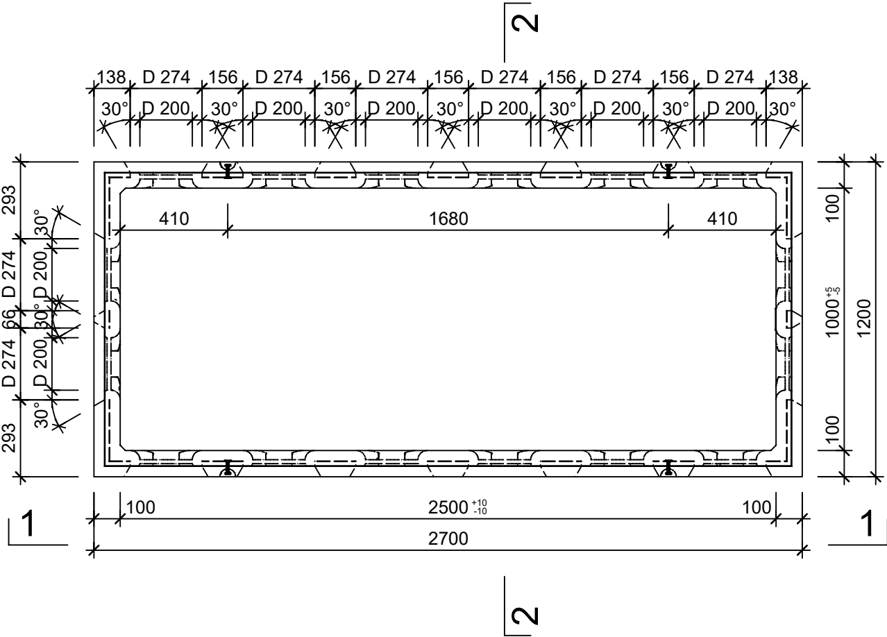
Grundriss, 1:20
