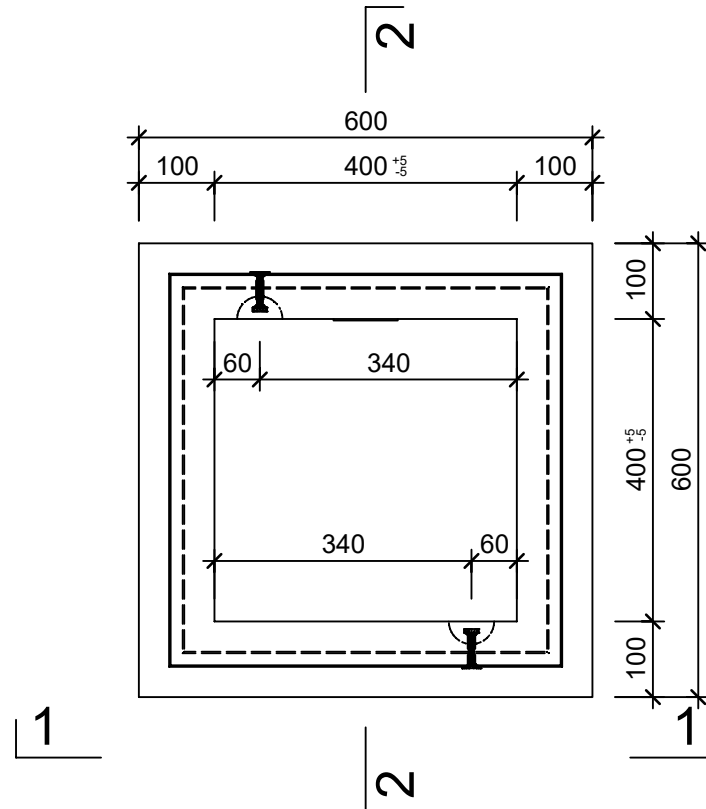
Grundriss, 1:10
