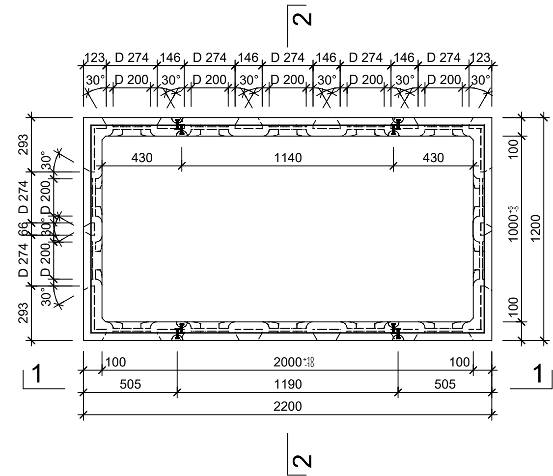
Grundriss, 1:20
