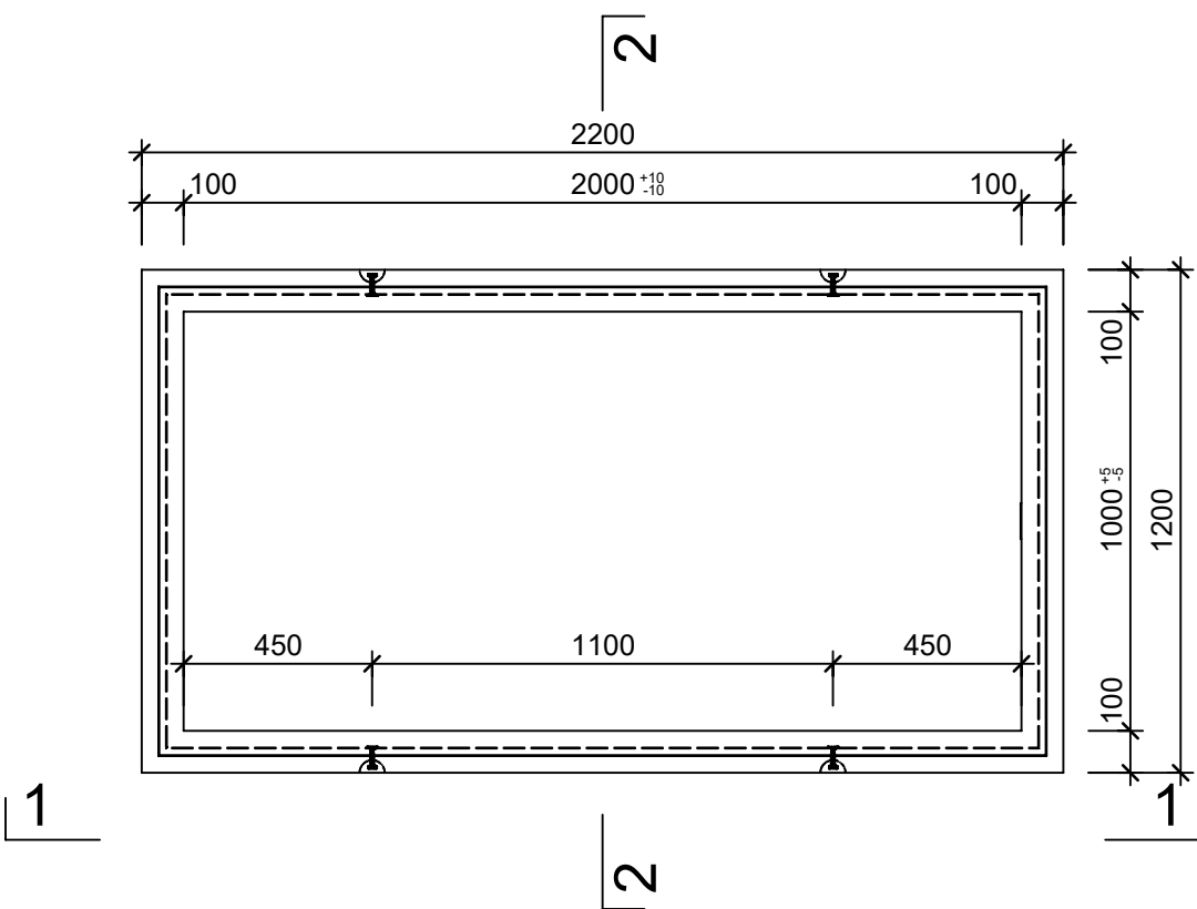
Grundriss, 1:20
