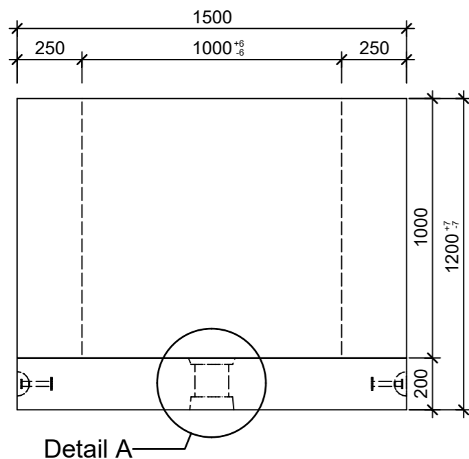
Schnitt 1-1, 1:20
