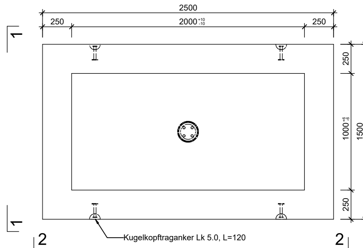
Grundriss, 1:20
