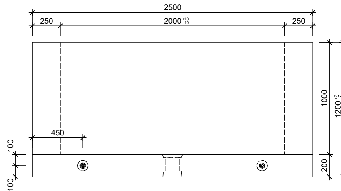
Schnitt 2-2, 1:20
