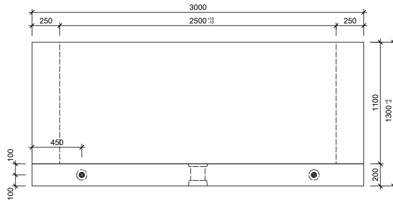
Schnitt 2-2, 1:20
