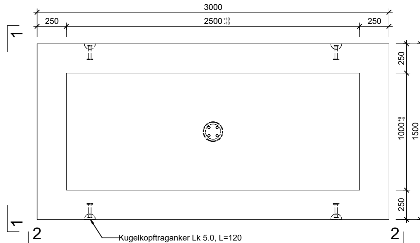
Grundriss, 1:20
