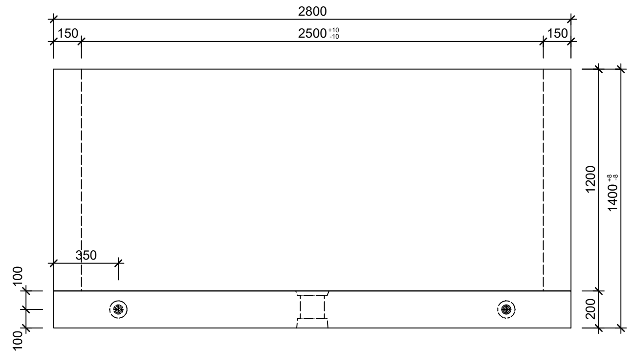
Schnitt 2-2, 1:20
