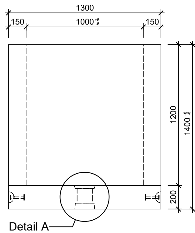
Schnitt 1-1, 1:20
