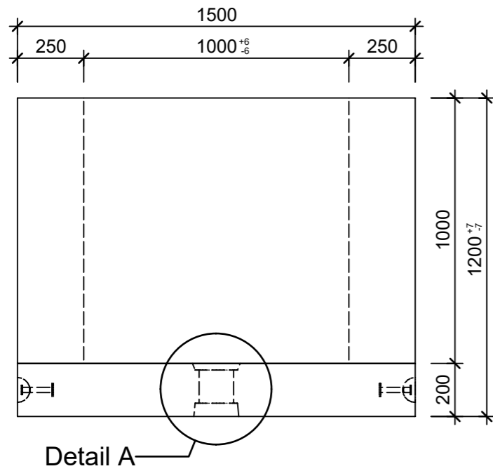
Schnitt 1-1, 1:20
