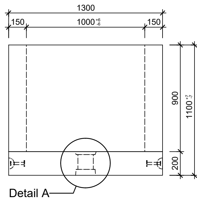
Schnitt 1-1, 1:20
