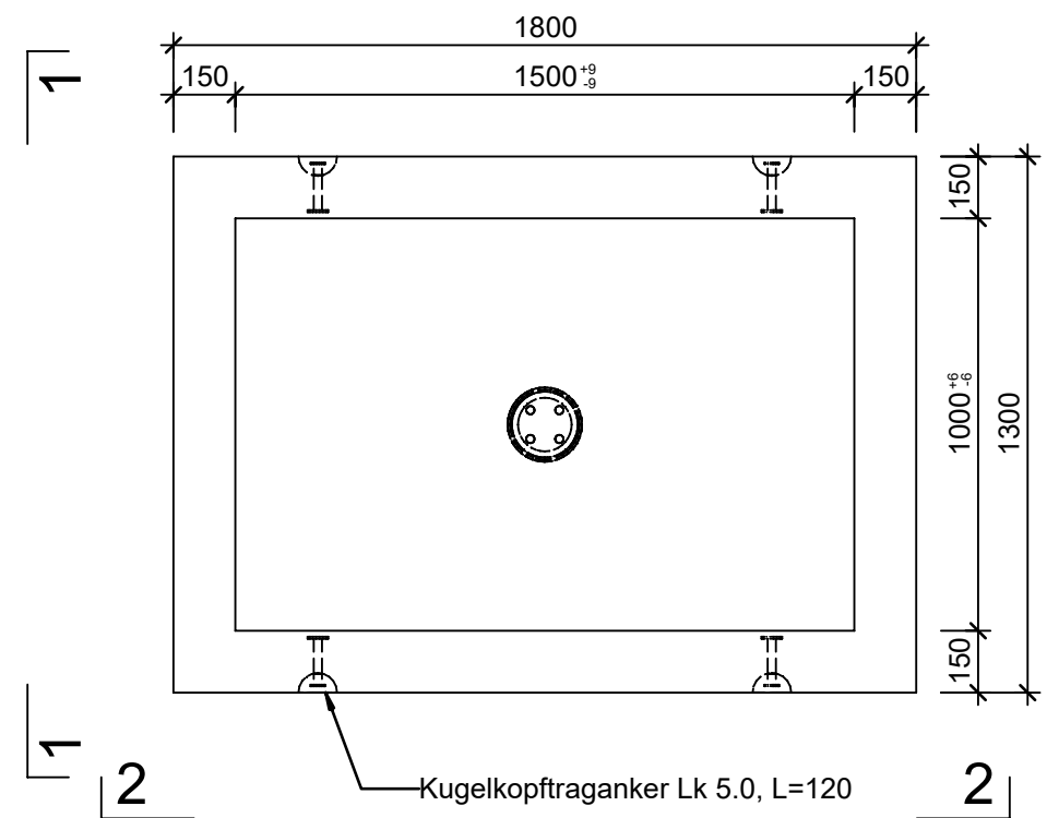
Grundriss, 1:20
