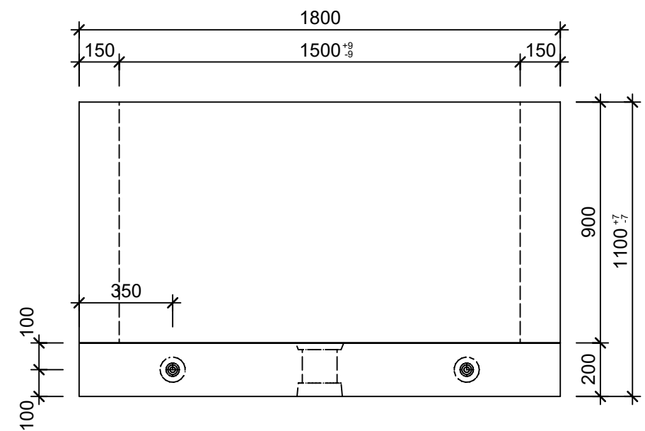
Schnitt 2-2, 1:20
