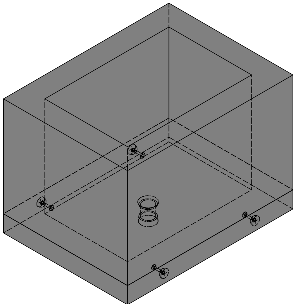
Isometrie, 1:20
