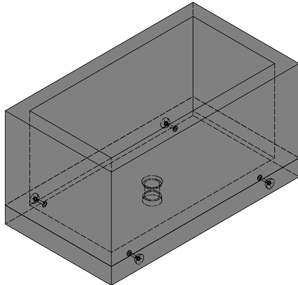
Isometrie, 1:20
