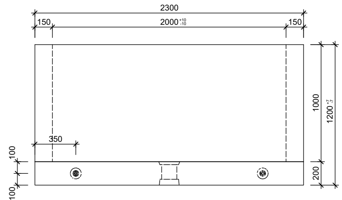
Schnitt 2-2, 1:20
