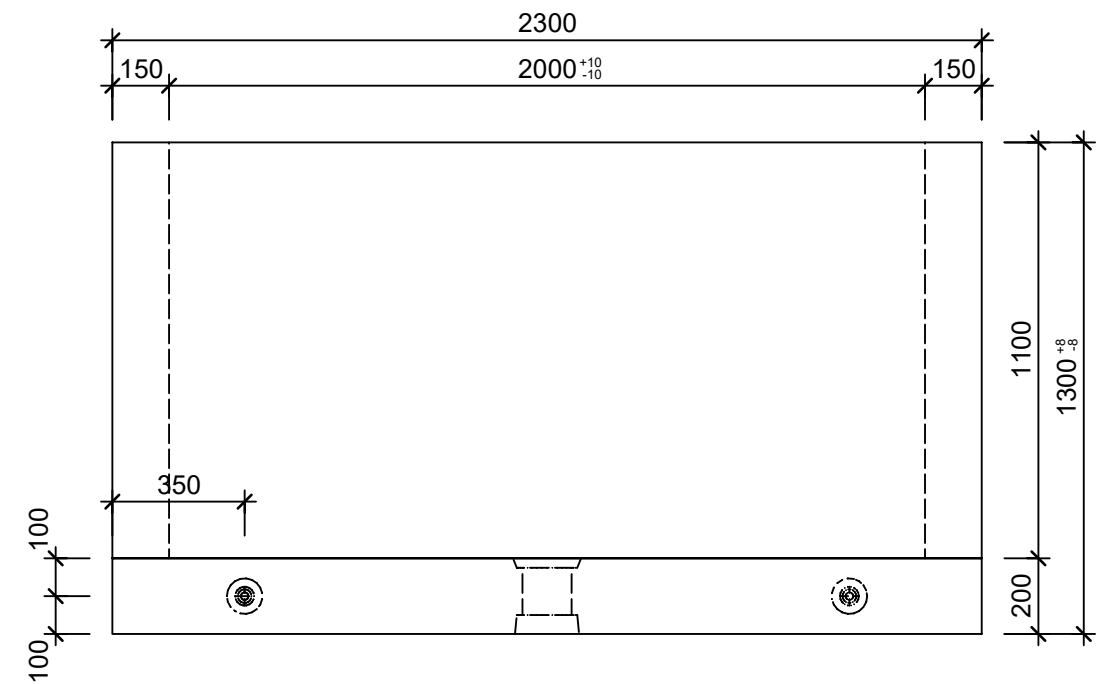
Schnitt 2-2, 1:20
