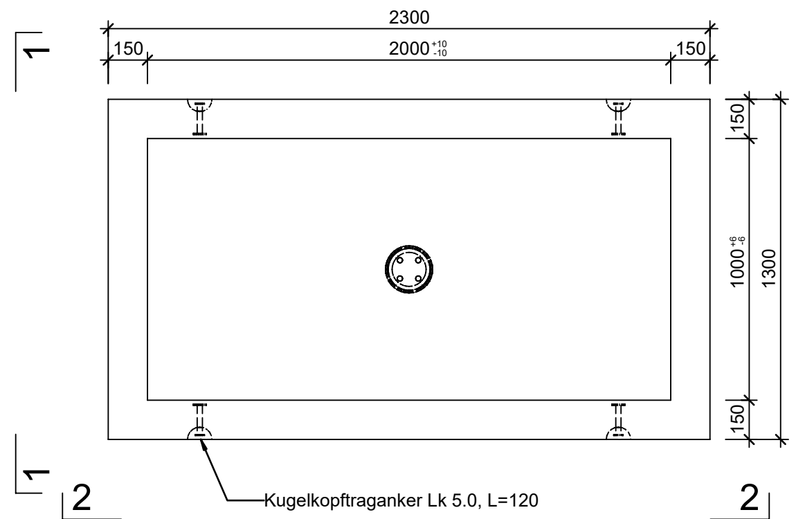
Grundriss, 1:20
