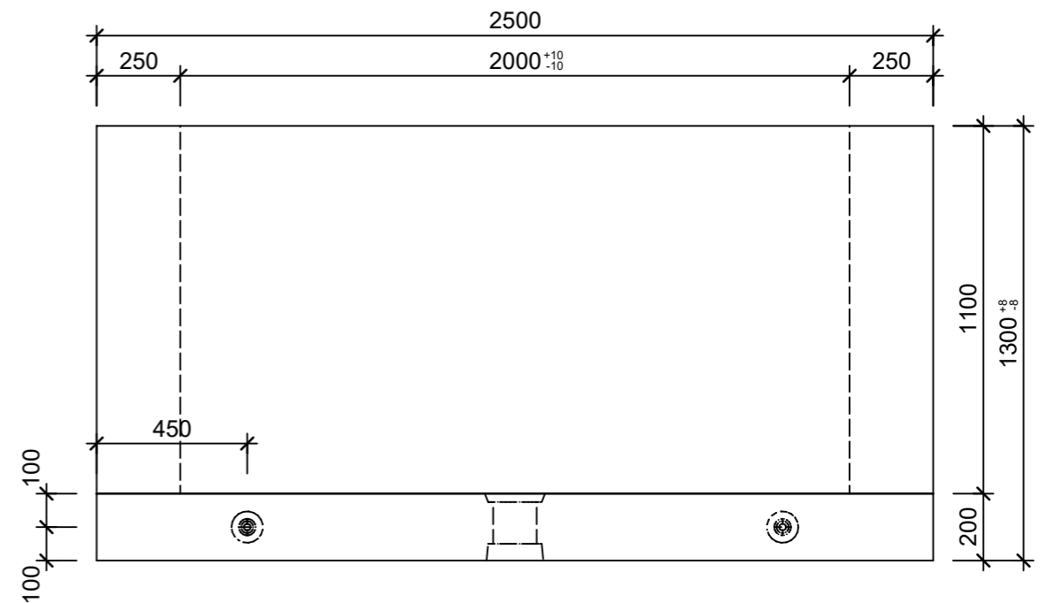
Schnitt 2-2, 1:20
