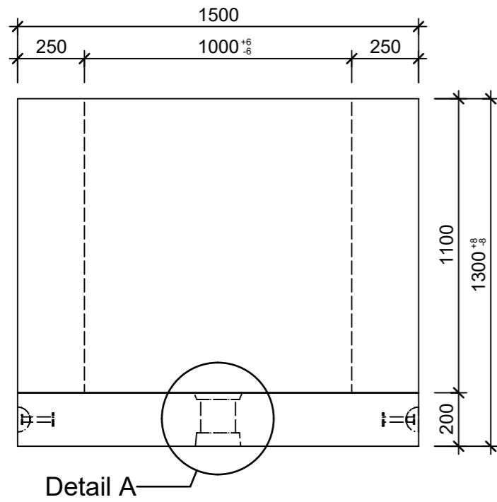
Schnitt 1-1, 1:20
