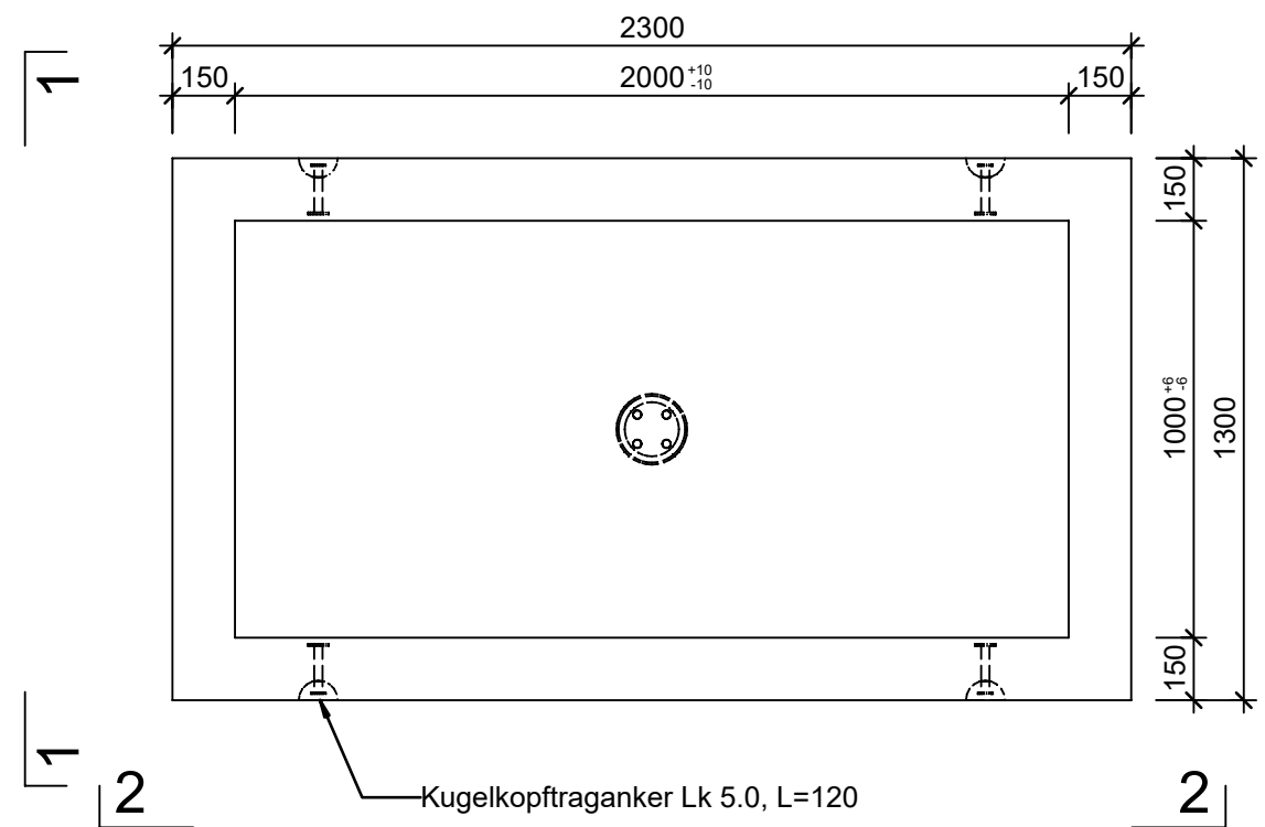
Grundriss, 1:20
