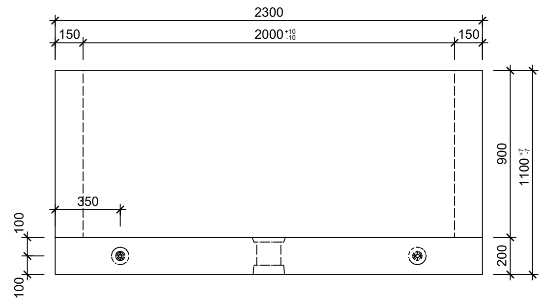
Schnitt 2-2, 1:20
