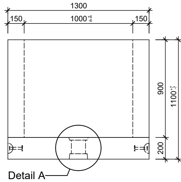
Schnitt 1-1, 1:20
