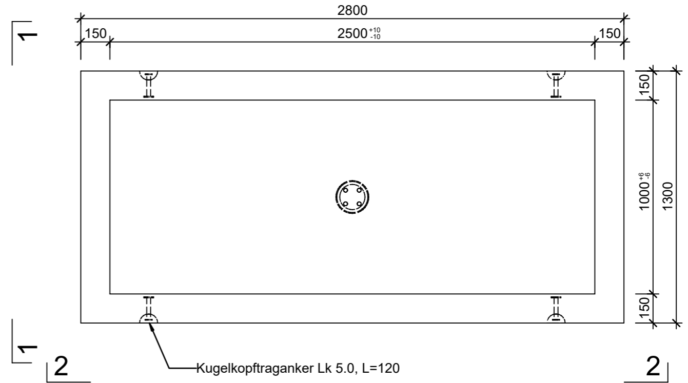
Grundriss, 1:20
