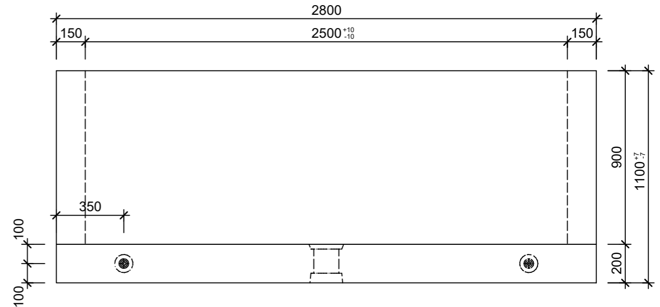
Schnitt 2-2, 1:20
