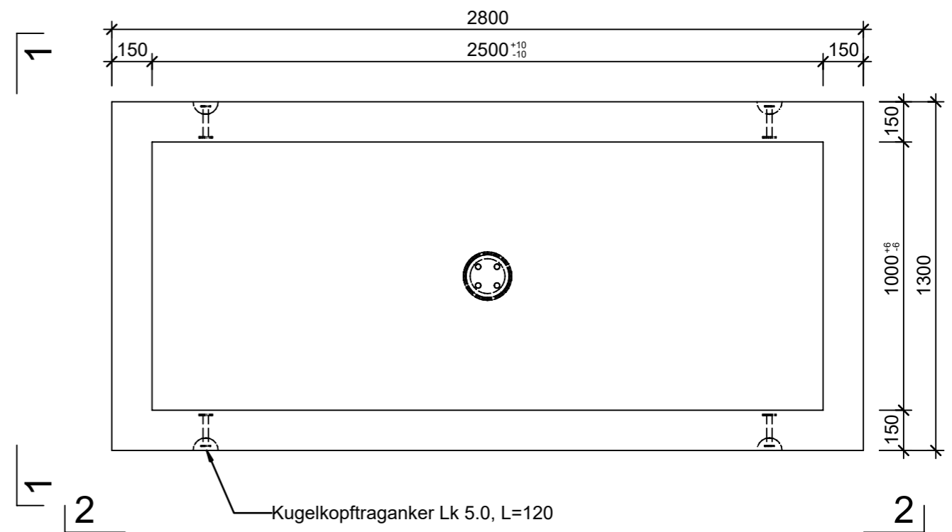
Grundriss, 1:20
