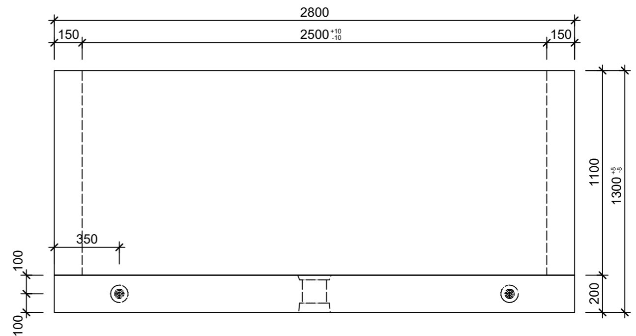
Schnitt 2-2, 1:20
