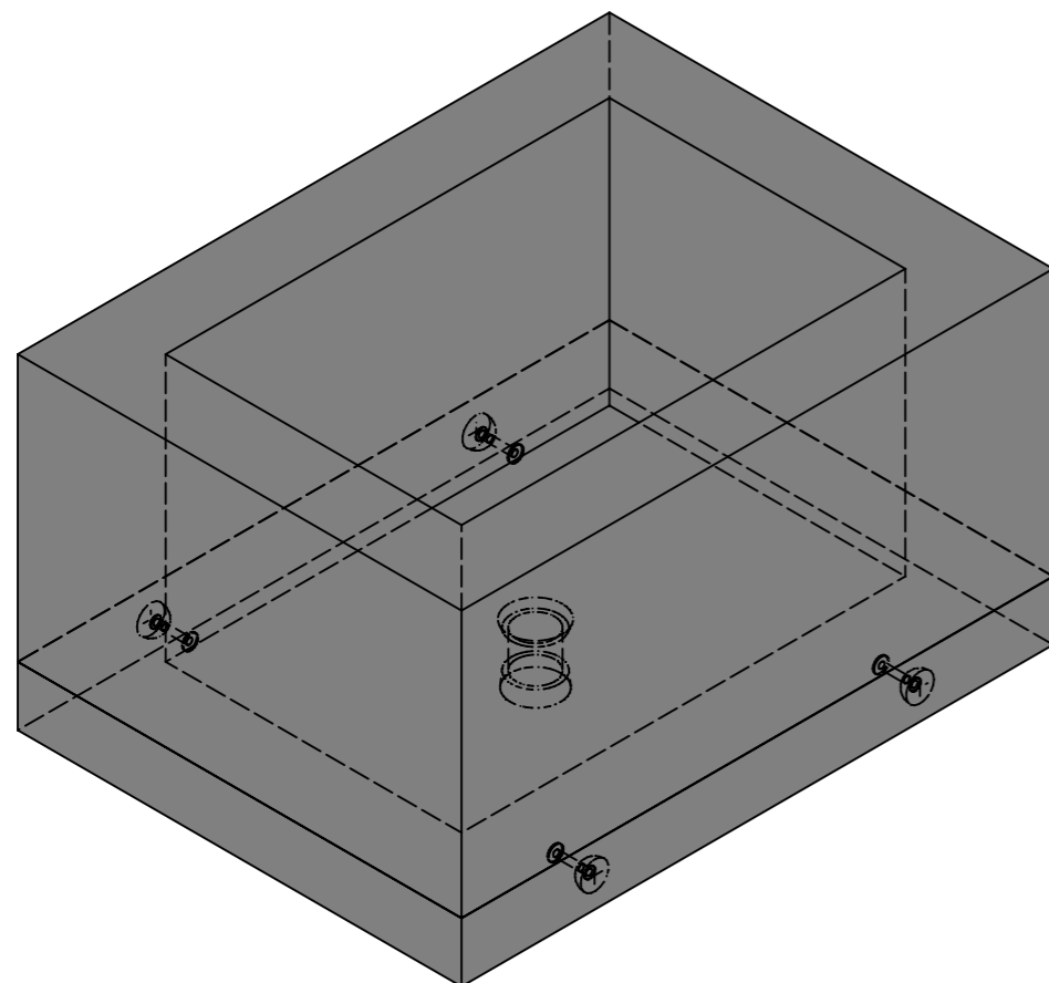
Isometrie, 1:20
