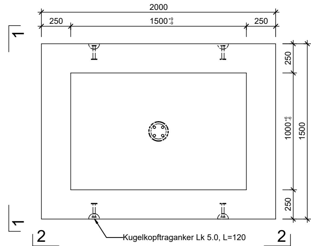
Grundriss, 1:20
