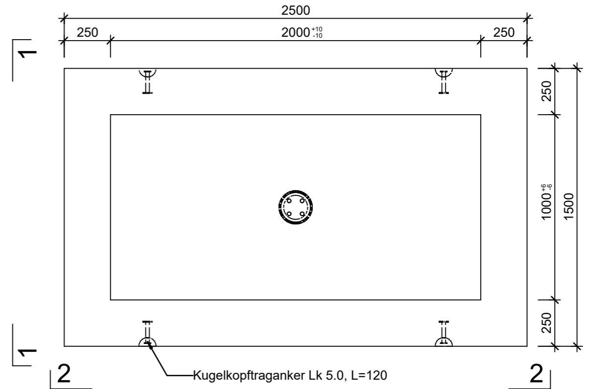
Grundriss, 1:20
