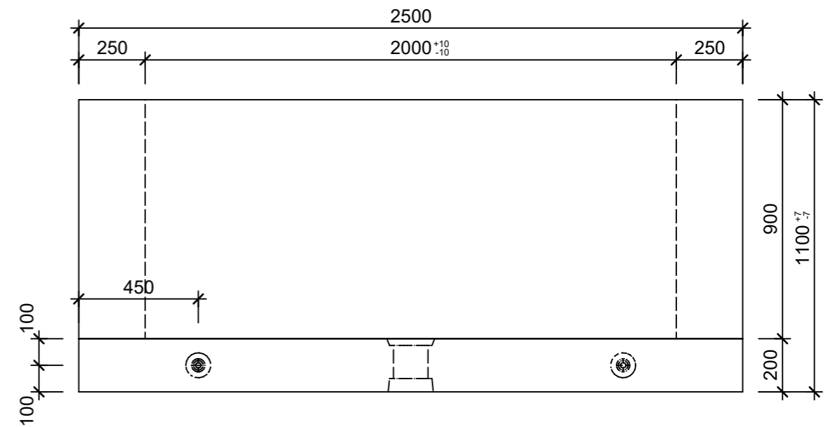
Schnitt 2-2, 1:20
