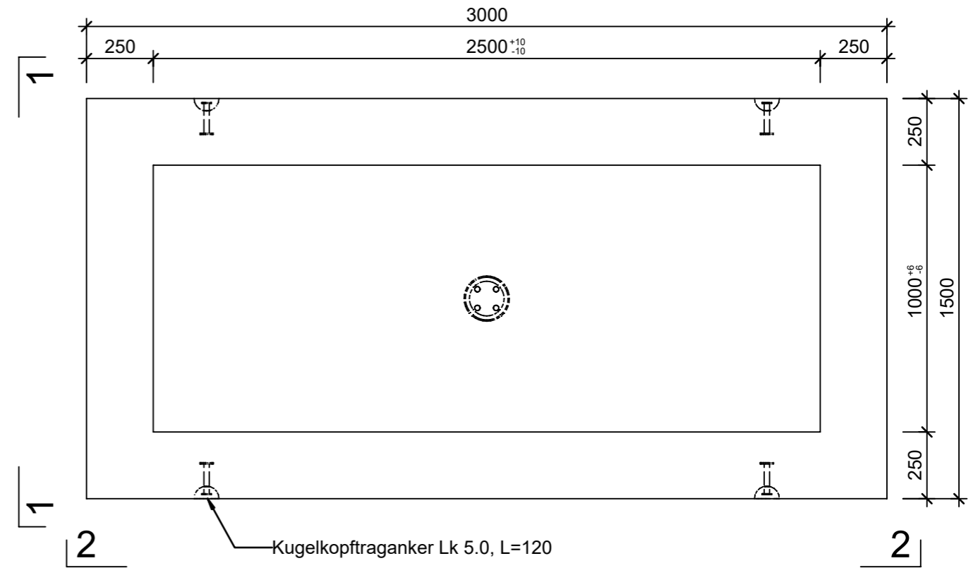
Grundriss, 1:20
