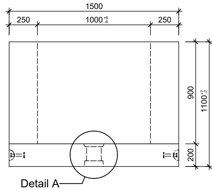
Schnitt 1-1, 1:20
