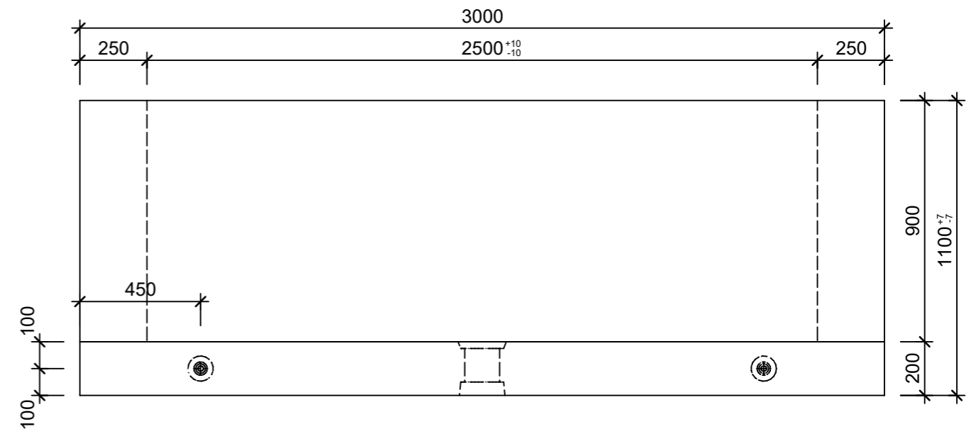
Schnitt 2-2, 1:20
