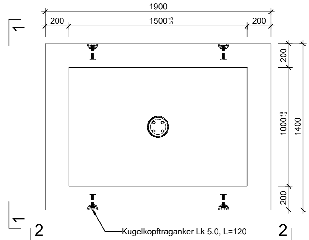
Grundriss, 1:20
