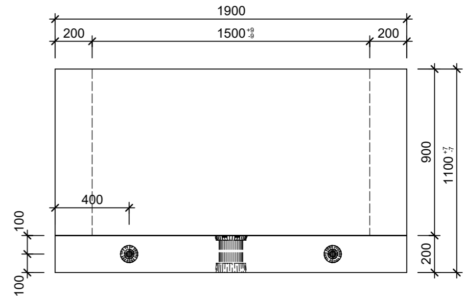
Schnitt 2-2, 1:20
