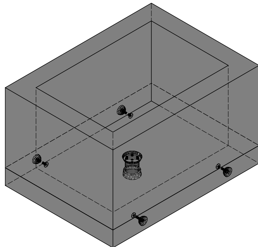
Isometrie, 1:20
