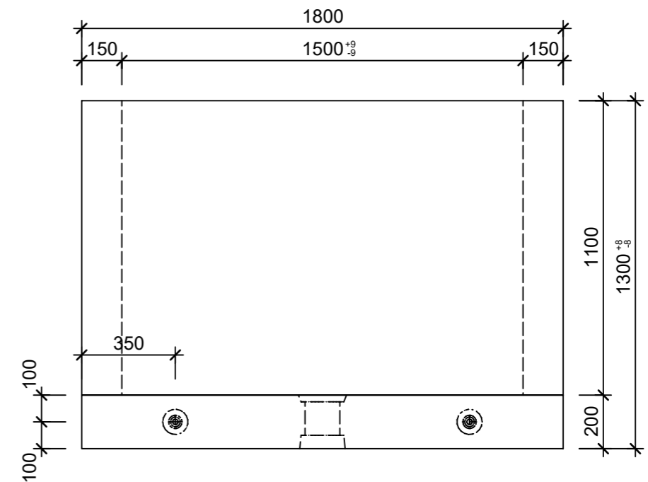
Schnitt 2-2, 1:20
