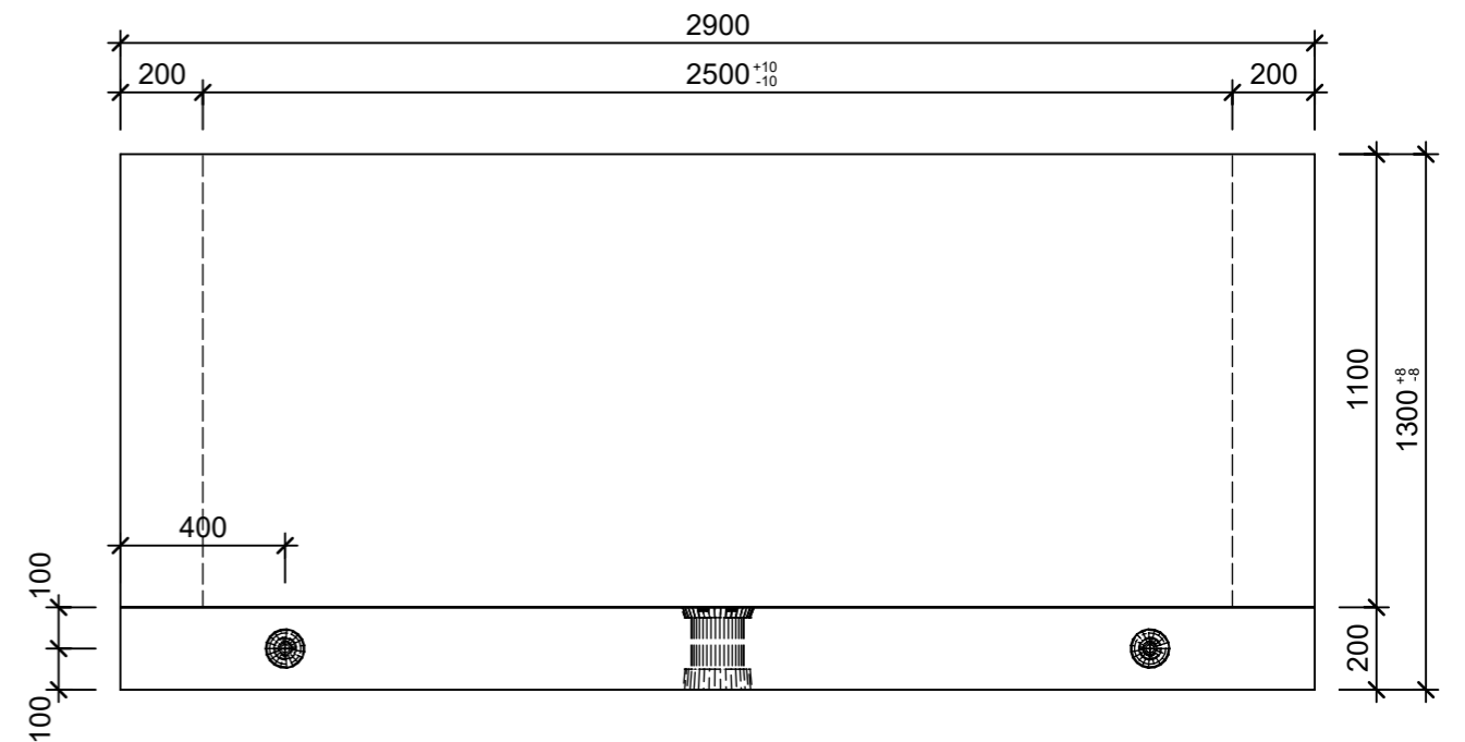
Schnitt 2-2, 1:20
