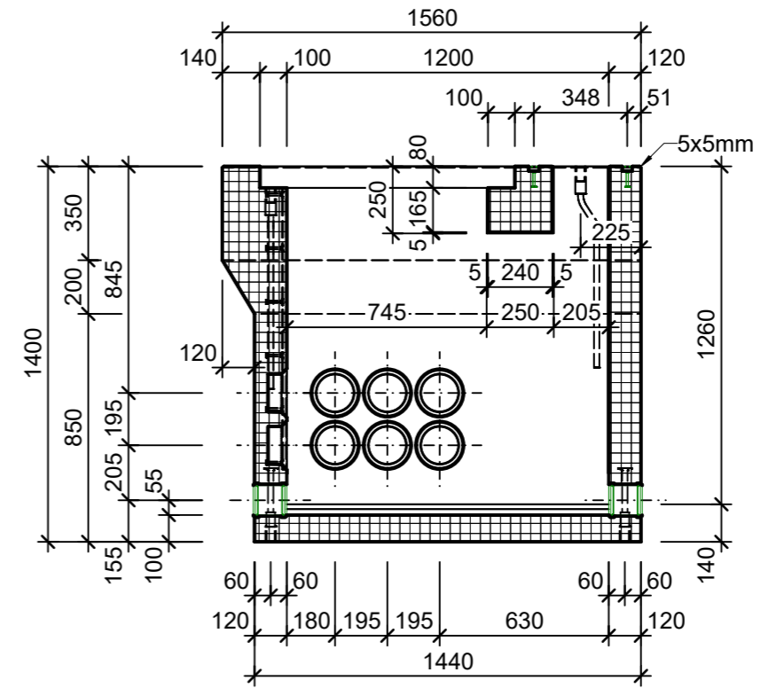
Schnitt 2-2, 1:25
