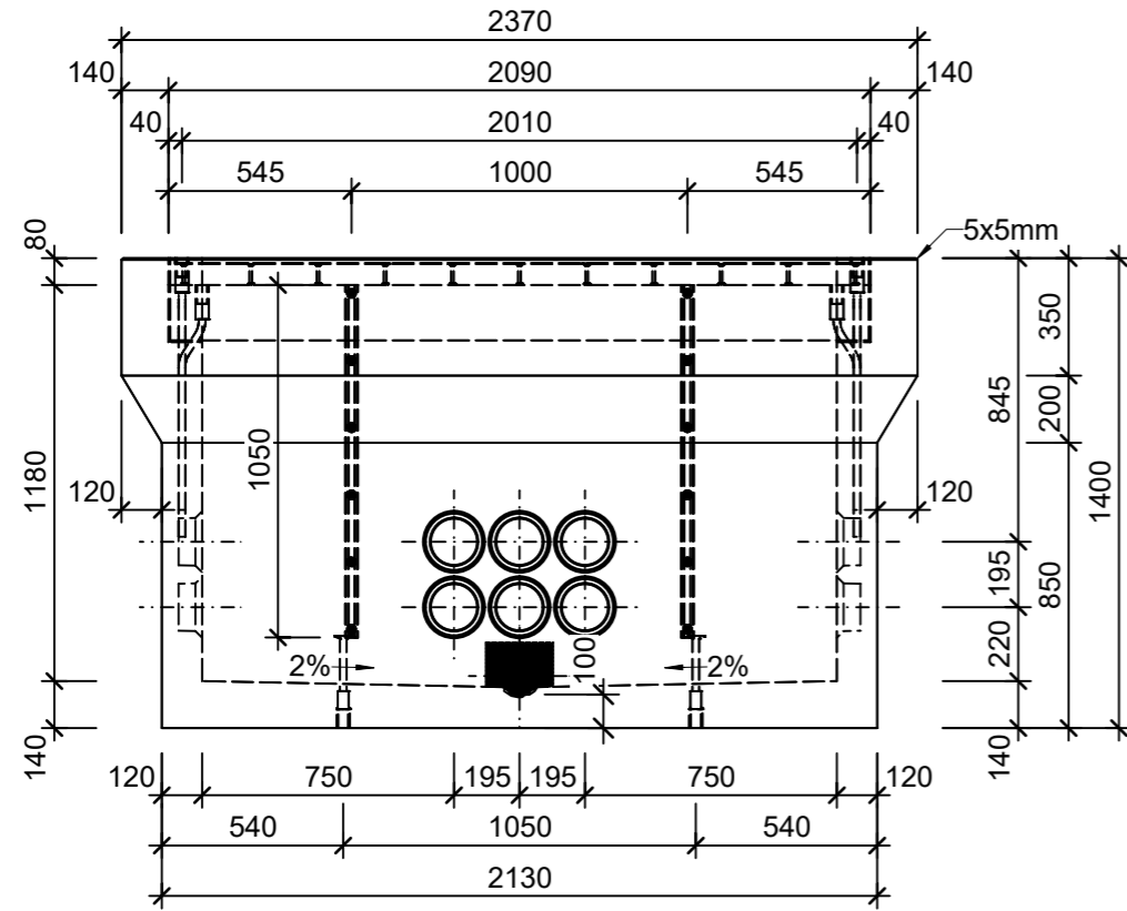
Ansicht 1-1, 1:25
