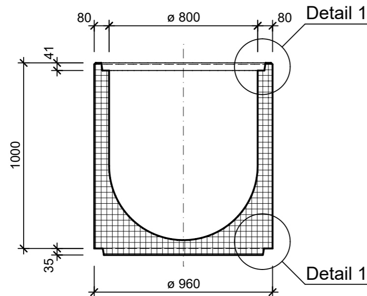
Schnitt A - A, 1:20
