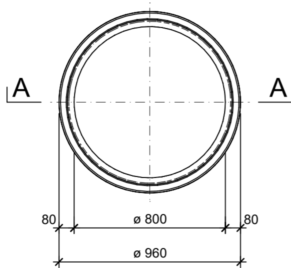
Grundriss, 1:20
