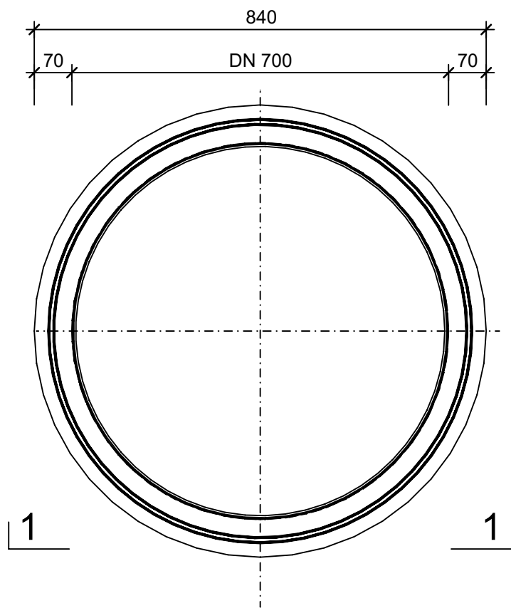
Grundriss, 1:10
