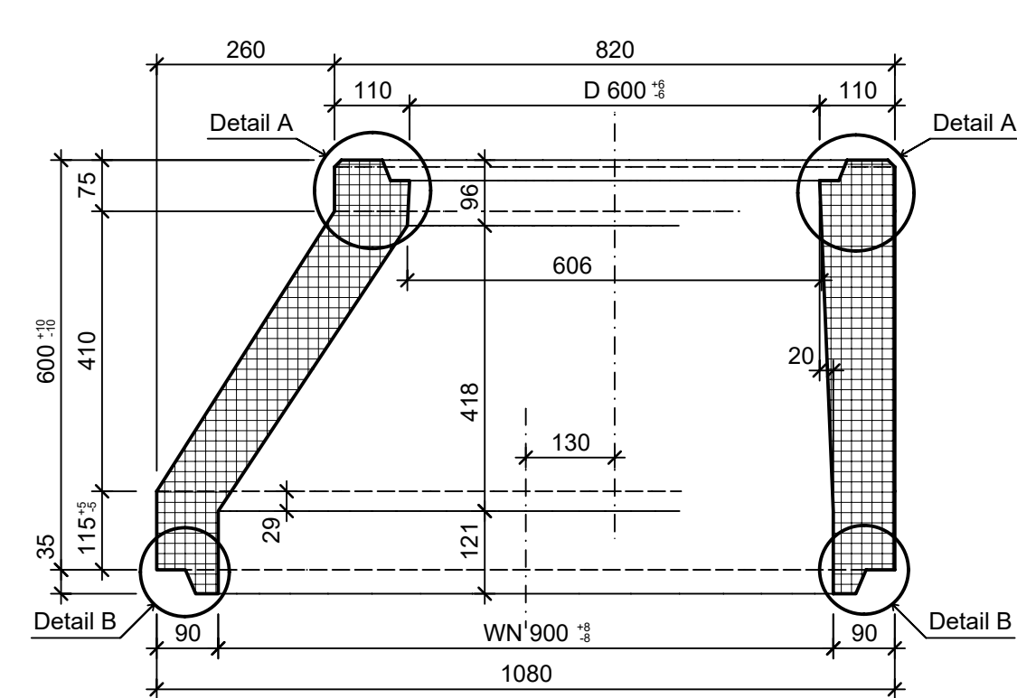
Schnitt 1-1, 1:10
