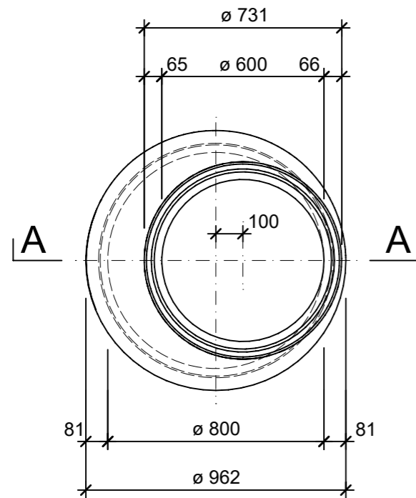
Grundriss, 1:20
