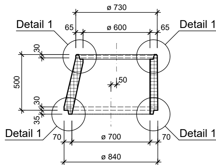
Schnitt A - A, 1:20
