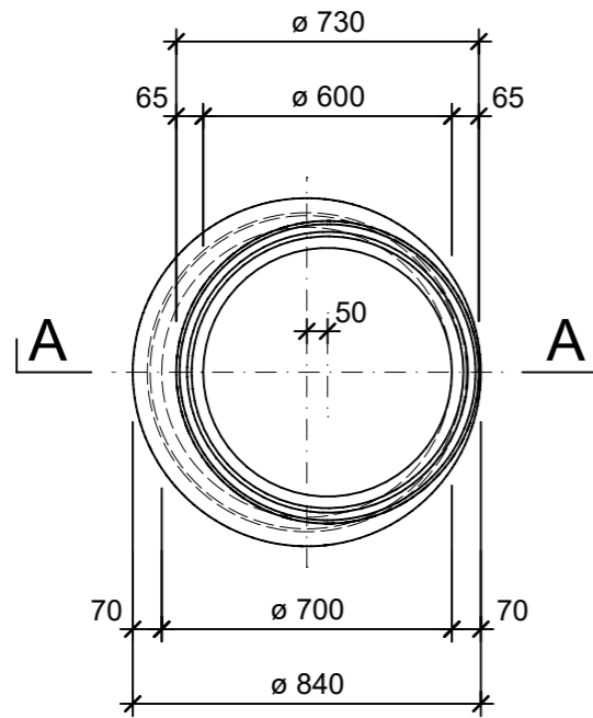
Grundriss, 1:20
