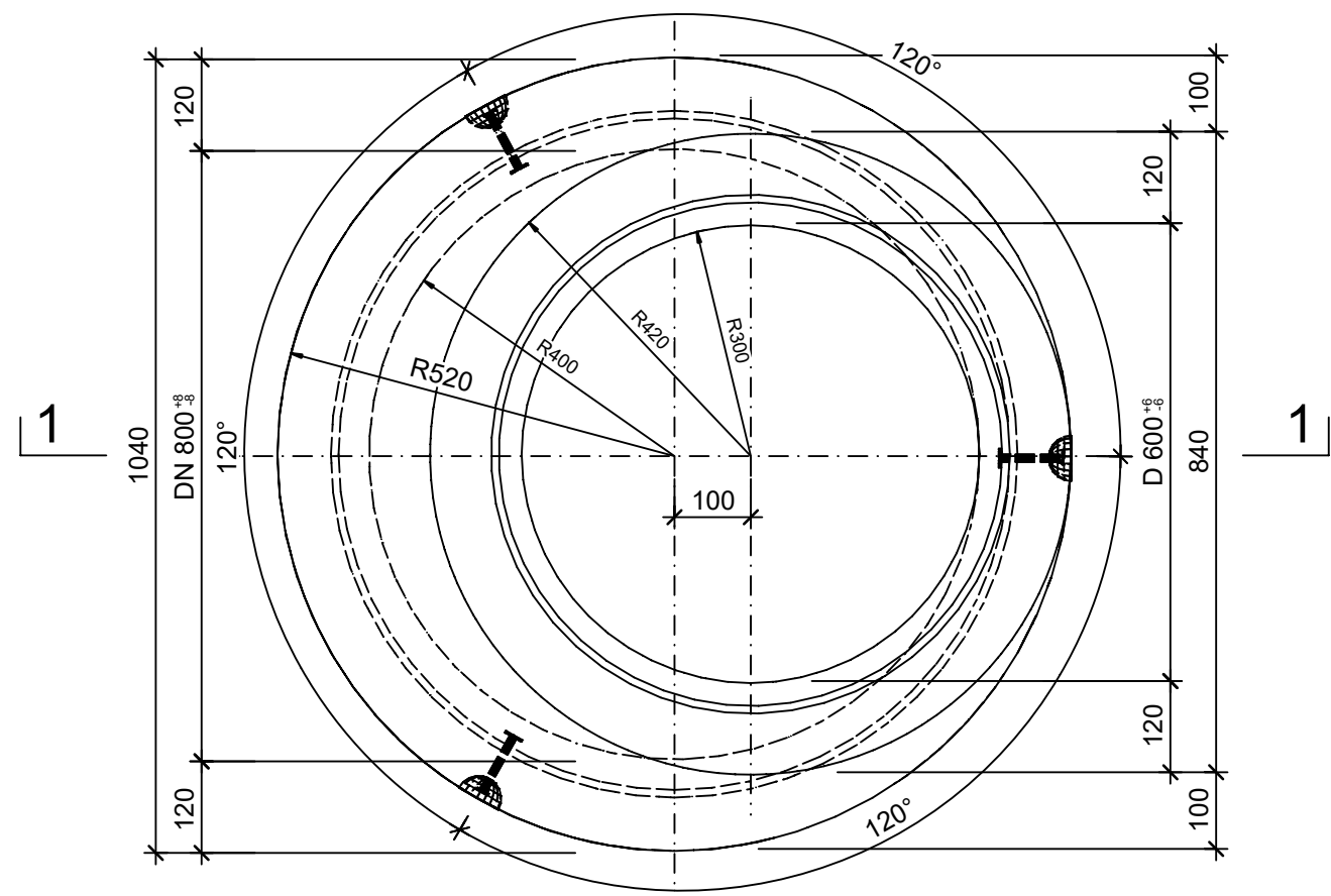
Grundriss, 1:10
